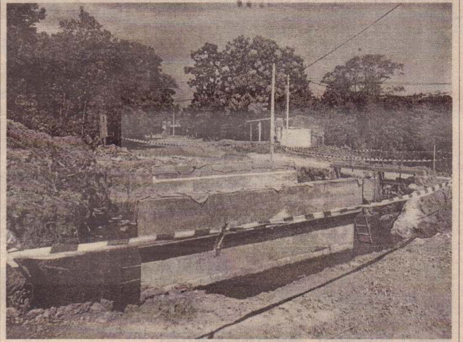
இரண்டாம் குளத்தின் நீர்ப்பாசன வாய்க்கால்கள் வட்டக்கச்சிப் பகுதியில் புனரமைக்கப்பட்டு வருகின்றன. (க-18)
