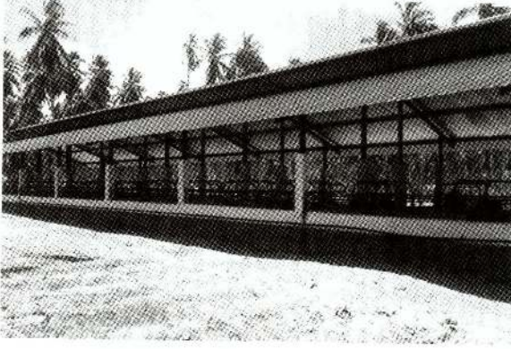
ஹொரக்கல பண்ணையில் நிருமாணிக்கப்பட்ட புதிய பன்றிக் கொட்டகை
