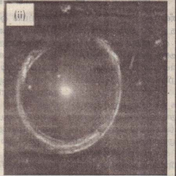
உரு 1: ஜன்ஸ்ஸின் ஈர்ப்பு வில்லைச் செயற்பாடு (I): திருப்பப்பட்ட விண்வெளி நேரம் (II) ஜன்ஸ்ஸின் ஒளி வளையம்
