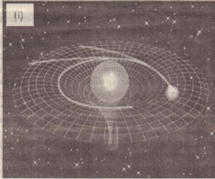
உரு 1: ஜன்ஸ்ஸின் ஈர்ப்பு வில்லைச் செயற்பாடு (I): திருப்பப்பட்ட விண்வெளி நேரம் (II) ஜன்ஸ்ஸின் ஒளி வளையம்
