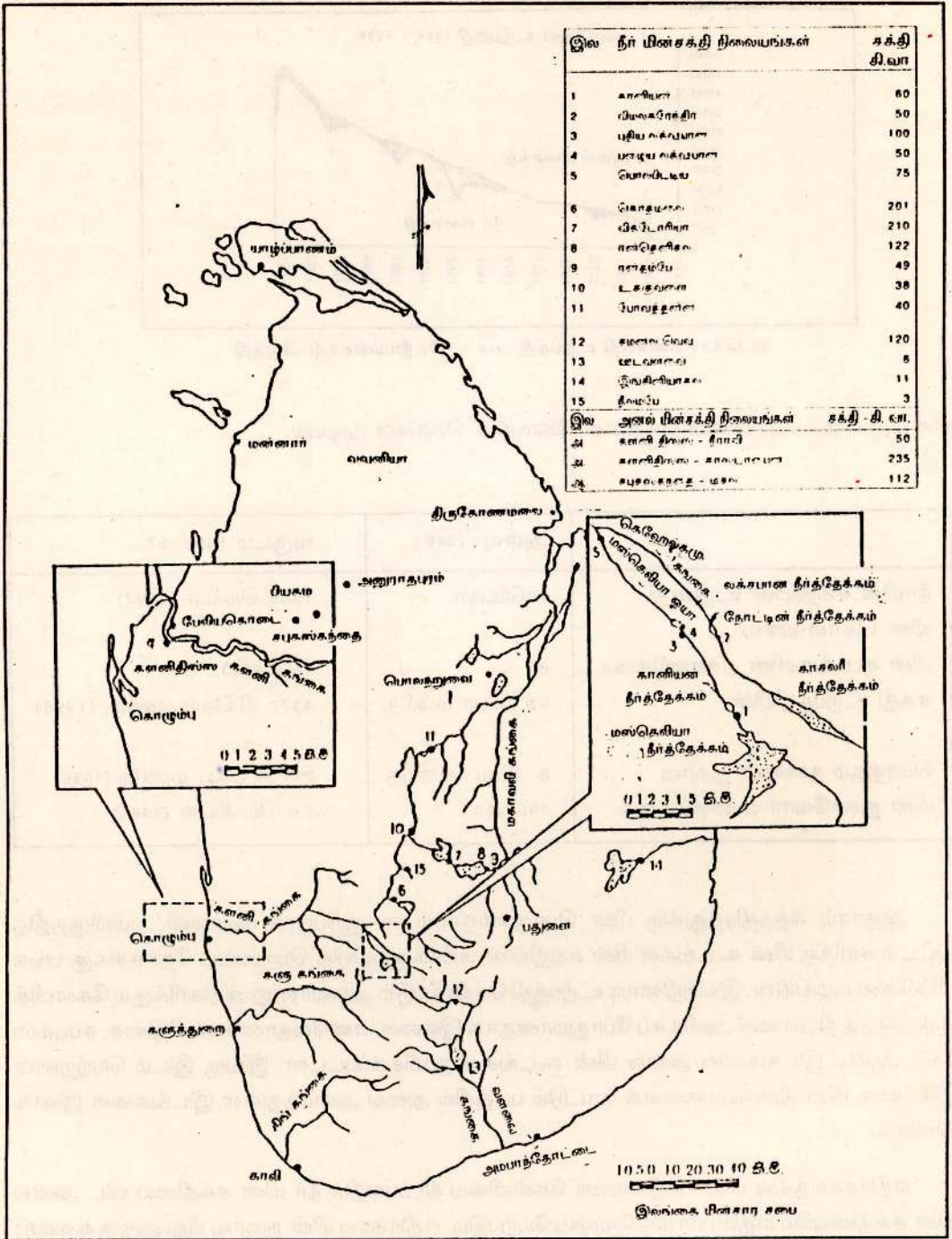
படம் 5.11 இலங்கையில் நீர் மின்சக்தி நிலையங்கள்
