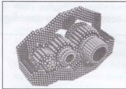
(15,342 அணுக்களாலான Parallel-Shaft speed reducer gear)
