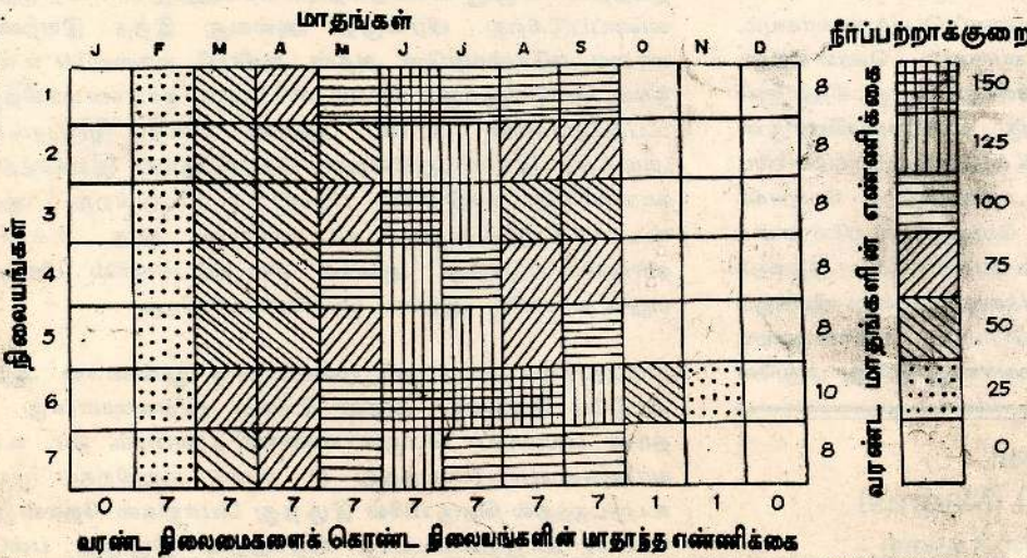
படம் 4: மாதாந்த நீர் பற்றாக்குறை நிலைமைகளின் அடிப்படையில் 7 நிலையங்களின் வறட்சித்தாயம்
