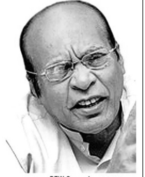
DEW Gunasekara
