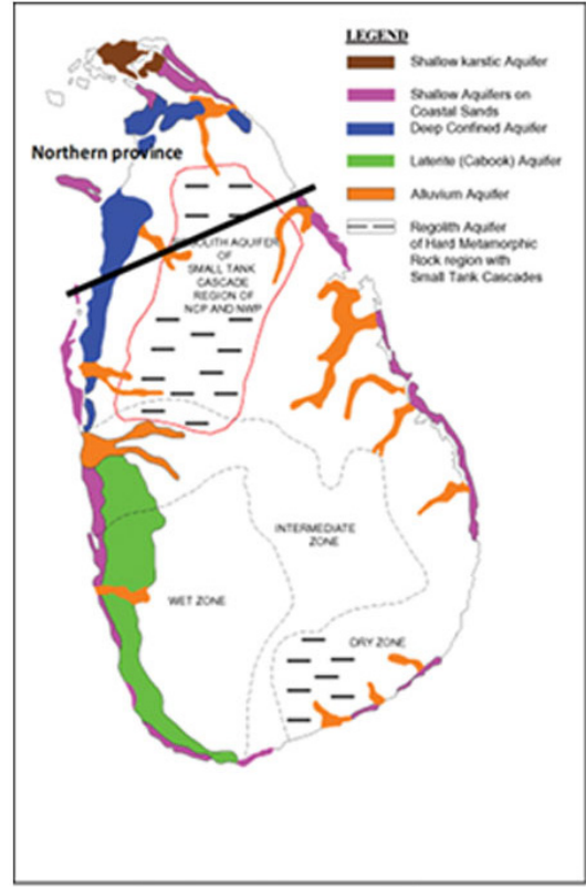
இலங்கையில் ஆறு முக்கியமான நிலத்தடிநீர்ப்பரப்புகள்
