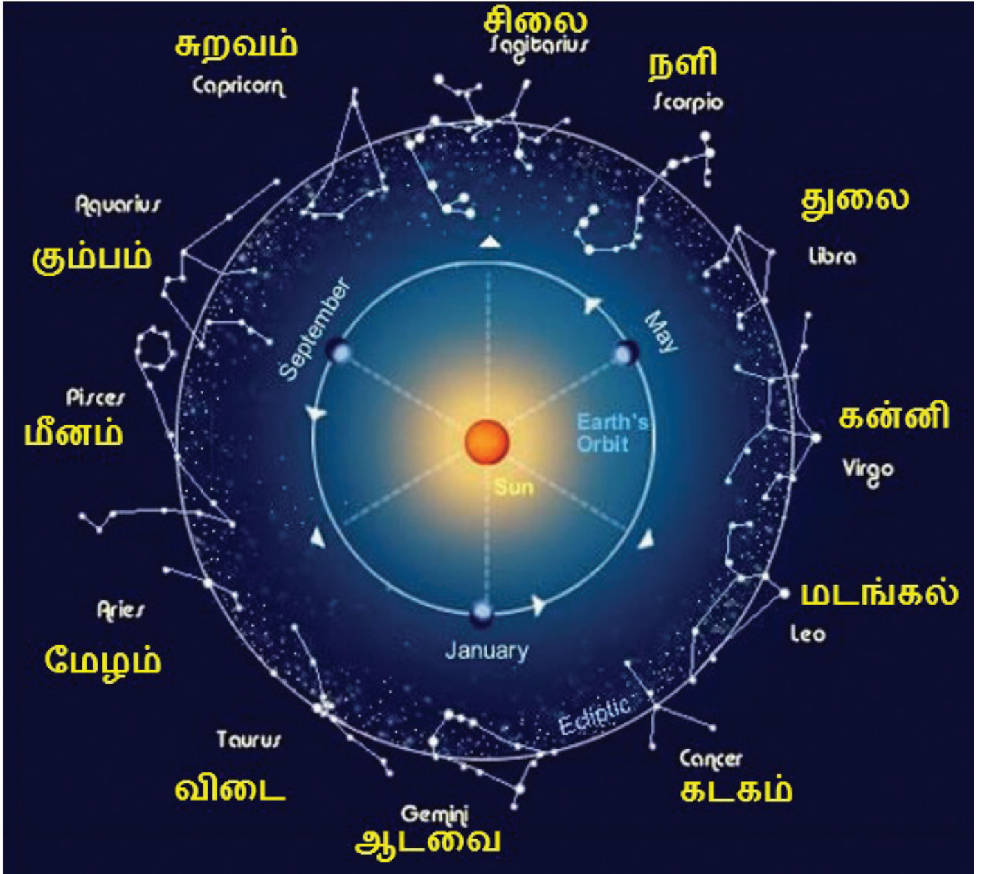
படம் 3: பன்னிரு ஓரைகள் அல்லது இராசி மண்டலங்கள் (12 Zodiacs Constellations) (இரா.சிவகுமார்.2023a).
