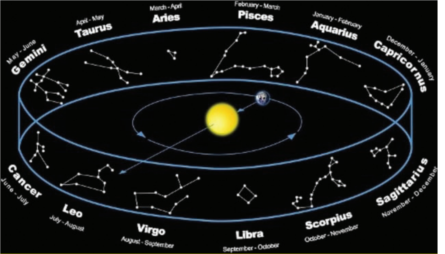
படம் 2: சூரியன் சிம்மம் / மடங்கல் (Leo) ஓரையில் எதிர்ப்படும் வெளித்தோற்ற நகர்ச்சி ( Sun's apparent motion against zodiac ).Thanks: (Star Constellations: The Zodiac> 2017)
