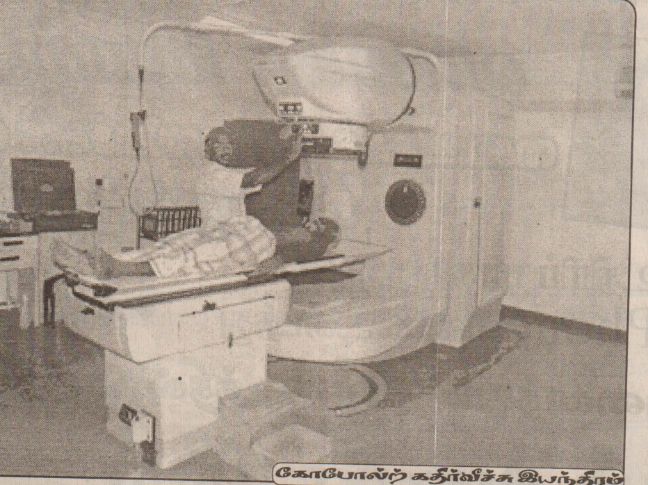
கோபோல்ட் கதிர்வீச்சு இயந்திரம்
