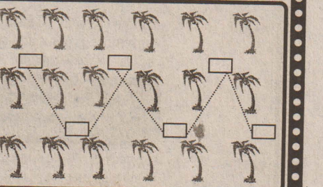
குறுகிய இடைத் தூரத்தில் நடுகை செய்யப்பட்ட தென்னை மரங்களுக்கிடையே, நான்கு தென்னைகளுக்கு நடுவில் குழிகளை அமைக்கலாம்.
