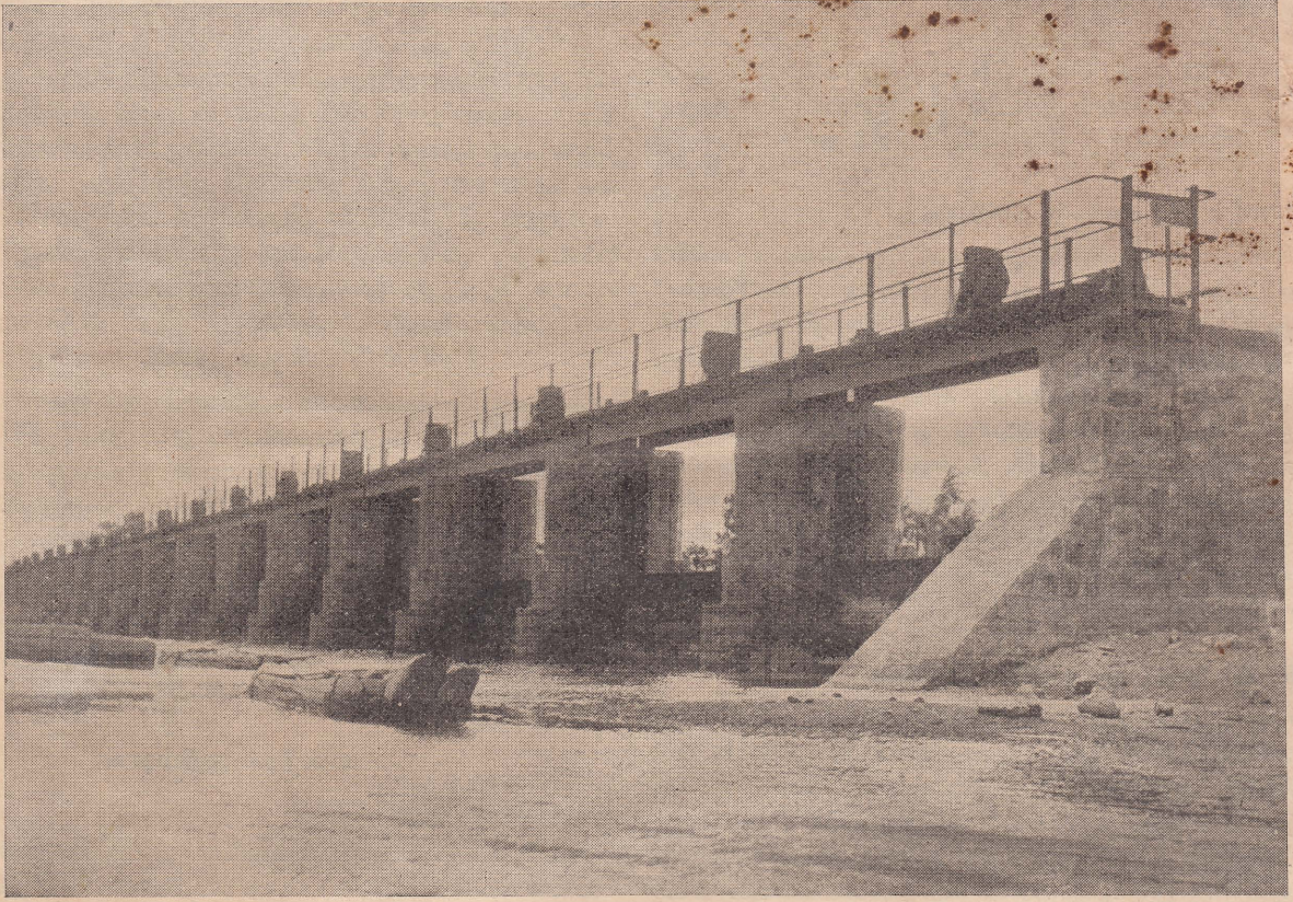
தொண்டமாற்று அணைக்கட்டு.
