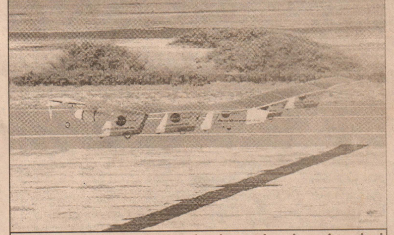
பகலில் சூரிய சக்தியாலும், இரவில் பட்டரி மின்சாரத்தாலும் பறக்கும் விமானத்தை அமெரிக்காவில் நாசா விண்வெளி ஆய்வு மையம் உருவாக்கியுள்ளது. ஹாவாய் தீவிலிருந்து இந்த விமானம் கடந்த 7 மீ திகழ் பறப்பட்டு. தொடர்ந்து 20 மணிநேரம் இந்த விமானம் பறக்கும் எனவும் நாசா விண்வெளி ஆய்வுமையம் கூறியுள்ளது.
