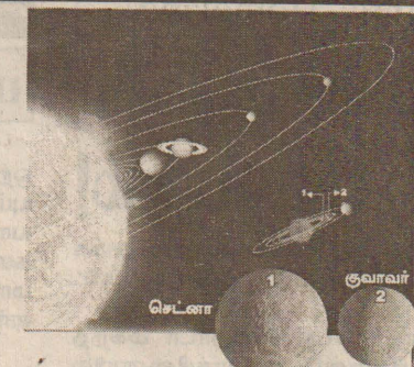
கான ஒளி ஆண்டுகளுக்கு அப்பால் உள்ள கிரகங்களின் தடவெப்ப நிலை, வளிமண்டலம் ஆகியவற்றைப் பற்றி அறிந்து கொள்ளக்கூடிய கருவி ஸ்பிடர்ஸ்பேஸ் தொலைநோக்கியில் உள்ள தென அவர் தெரிவித்தார்.
