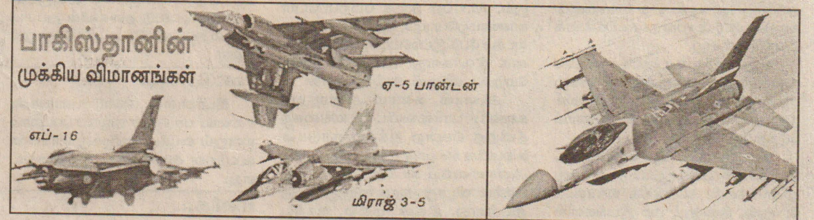
பாகிஸ்தானின் முக்கிய விமானங்கள் ஏ-5 பாண்டன், எப்-16, மிராஜ் 3-5
