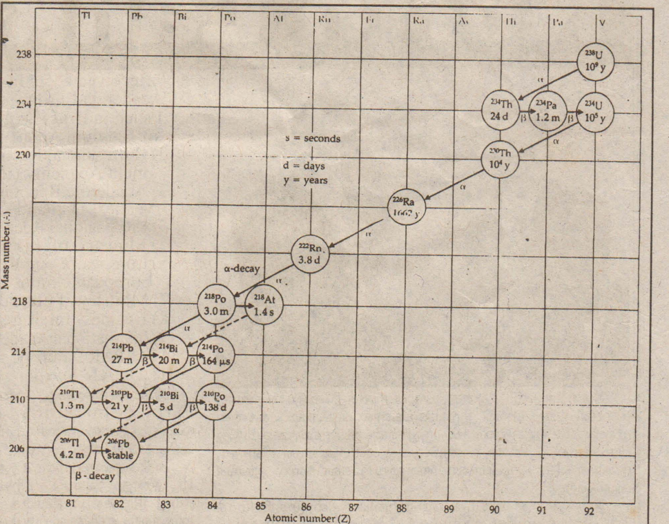
U-238 இல் இருந்து Pb - 206 ற்கான கதிர் தொழிற்பாட்டுத் தொடர்
