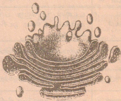
கொல்கியுடலின் முப்பரிமாண அமைப்பு
