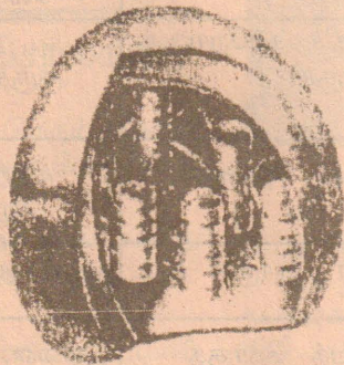
பச்சையலுருமணியின் முப்பரிமாண அமைப்பு
