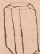
ஒரு சரிவுக் கந்தகம்
