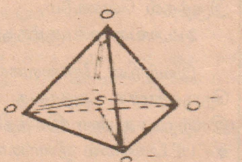
\text{SO}_2 இன் மூலக்கூற்றுருவம்
