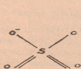
\text{SO}_2 இன் கட்டமைப்பு
