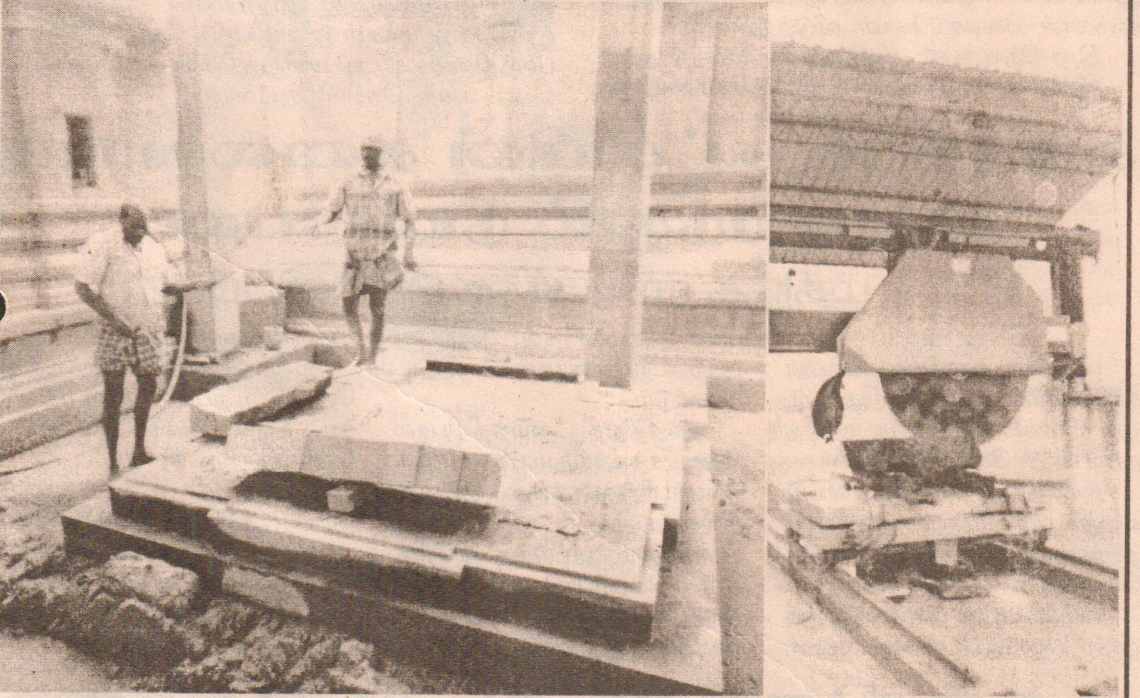
காரைநகர் துறைமுக சீத்திர கூட சீத்திவிநாயகர் ஆலயம் புத்தாக கருங்கல்லினால் அமைக்கப்பட்டுவருகிறது. பாரிய கியந்திரங்களின் உதவியுடன் நிர்மாணப்பணிகள் இடம்பெற்று வருவதைக் காணலாம். (50)
