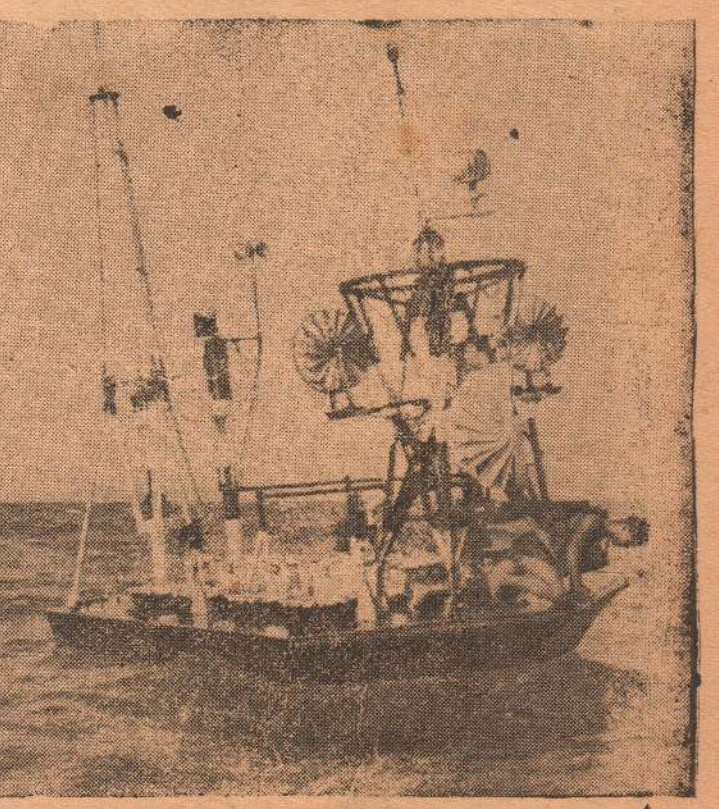
100 கிலோ மீட்டர் பரப்பு தண்ணீர் புறத்திலுள்ள கால நிலையை அளந்து தெரிவிக்கவல்ல உபகரணக் கப்பல் ஒன்று மெக்ஸிக்கோ குடாவில் நங்கூரமிட்டு நிறுவப்பட்டுள்ளது. 'நோமாத்' என்று அழைக்கப்படும் இந்த உபகரணம் ஆட்களின் உதவியின்றித் தானாகவே தொழிலாற்றாமாம், தண்ணீர், காற்று ஆகியவற்றின் உஷ்ண நிலையையும் காற்றின் வேகம், திசை ஆகியவற்றையும் நீரோட்டங்களின் திசைகளையும் இந்த உபகரணம் அறிவுறுத்தும்.
