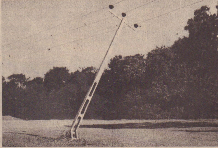
மிகவும் ஆபத்தான நிலையில் முற்றாக முறிவடைந்து மின் கம்பிகளில் தாங்கியவாறு A35 வீதி புதுக்குடியிருப்பு பொலிஸ் நிலையத்திற்கு அண்மையாக காணப்படும் மின் கம்பத்தை படங்களில் காணலாம். (படங்கள்- நெட்பானா செய்தியாளர்)
