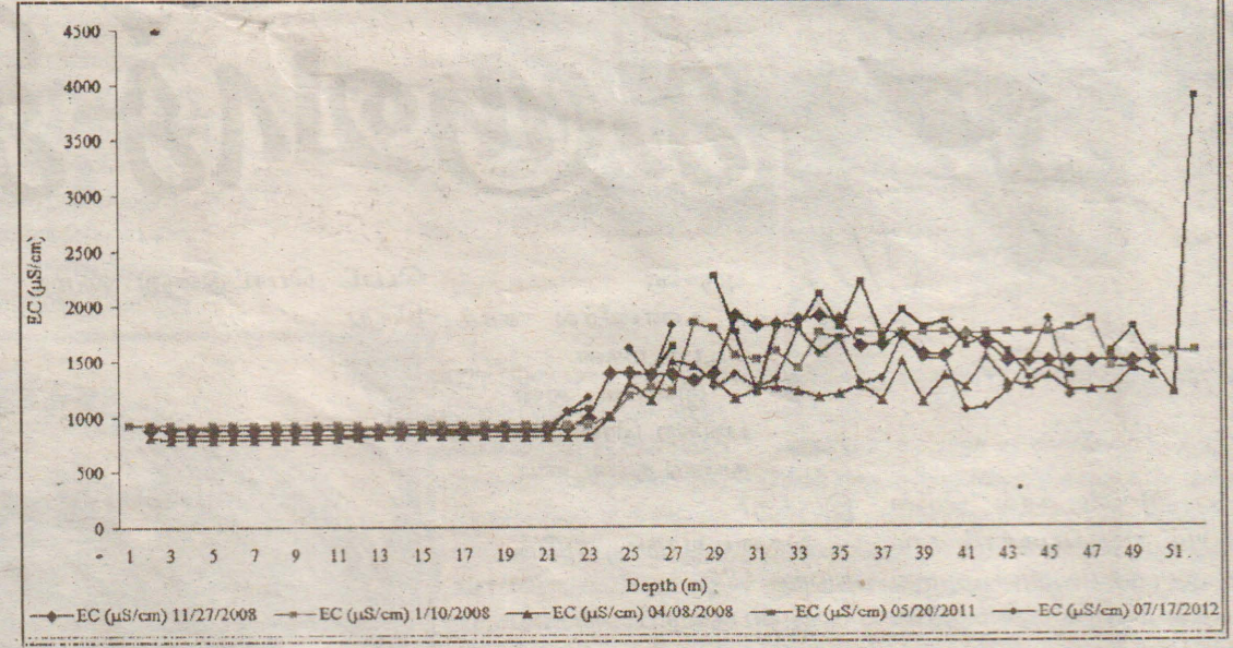
படம் - 03: நிலாவரைக் கிணற்றின் ஆழத்துடனான மின்கடத்து திறனின் மாற்றம்.
