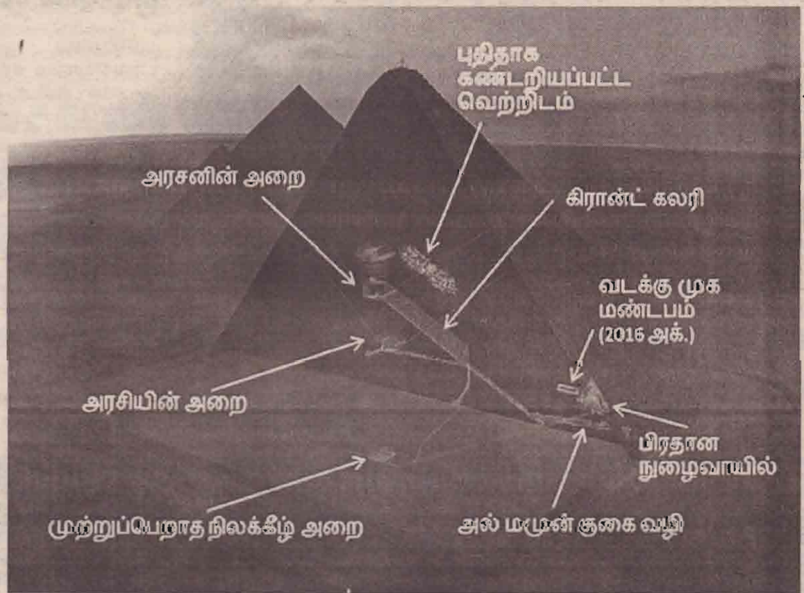
பிரமிட்டின் உட்கட்டமைப்பு (பயன்படுத்தப்பட்டுள்ள படமானது (Scan Pyramids Mission) இனால் உருவாக்கப்பட்டதாகும்)
