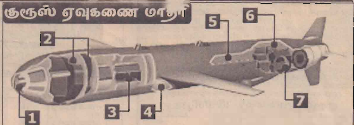
குருஸ் ஏவுகணை பகுதிகள் 1. புற உதகக் கதிர்களைக் கொண்டு விம்பங்களை உணரும் கருவி, (infrared imagery sensor), 2. கிலக்குகளை வழிகாட்டும் அமைப்பு, (guidance system), 3. வெடிக்குண்டுக் கட்டிப்படுகு பகுதி (warhead), 4. எதிரியின் நிலைகளை மீளும்புள்ள படங்கள் மூலம் வெளிப்படுத்தும் டிஜிட்டல் கருவி, (digital scene matching illuminator), 5. பிரதான என்ஜின் தாங்கி, (main fuel tank), 6. யுகோ அமைப்பைக் கொண்டு நிலைமைகளை ஒப்பிட்டு அமைப்பு, (terrain matching system) 7. ஒலியின் வேகத்தில் செல்லக்கூடிய 'டேர்போ ஷெட்' கியூட்டிர்ம், (turbojet subsonic engine)
