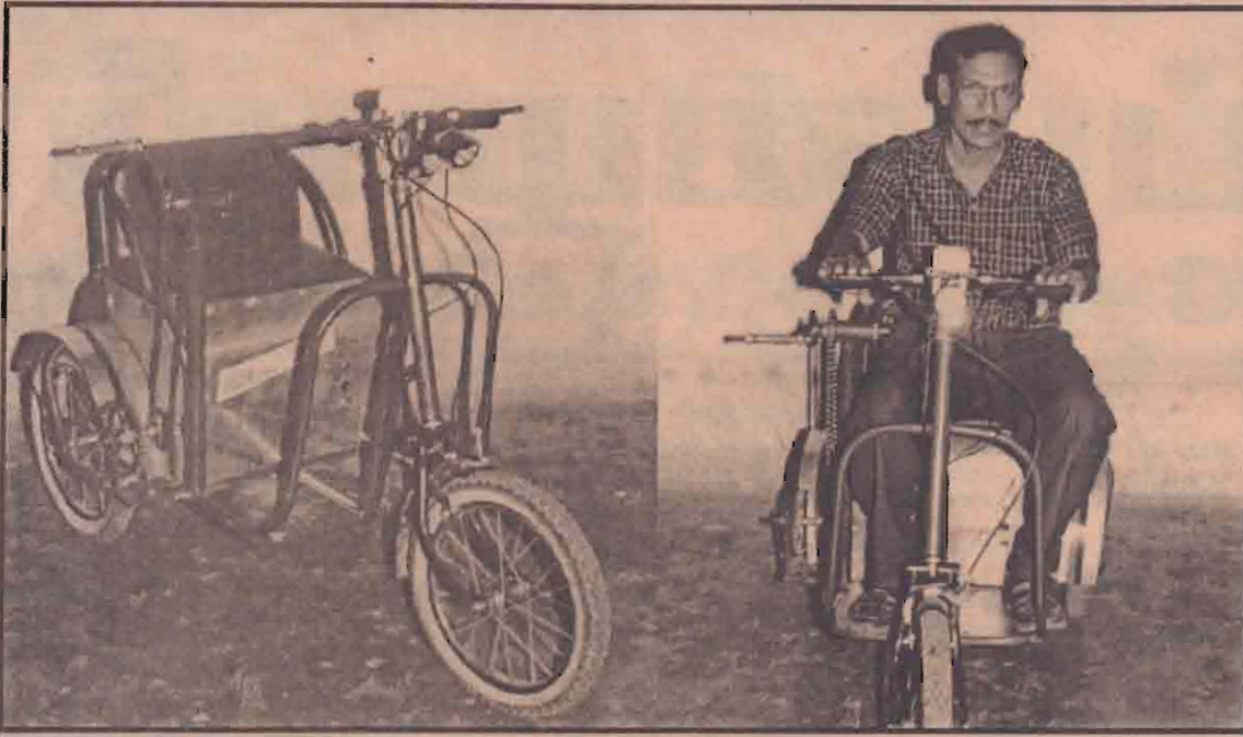
ஜெயப்பூர் நிறுவனத்தின் யாழ்ப்பாண முகாமையாளர் பா.மகேந்திரகுமாரினால் வலுவிறந்தகோரின் பாவனைக்கென முதன்முதலாகத் தயாரிக்கப்பட்ட பற்றியில் கியங்கக்கூடிய முச்சக்கர மோட்டார் வண்டியினை முதலாவது படத்தில் காணலாம். மணிக்கு 15 கிலோமீற்றர் வேகத்தில் செல்லக்கூடிய கிவ்வண்டியை பா.மகேந்திரகுமார் கியங்க வைப்பதை கிரண்டாவது படத்தில் காணலாம். மேற்படி முச்சக்கர மோட்டார்வண்டி கையினாலும் கழற்சிச் செலுத்திச் செல்லக் கூடியதாகவும் அமைக்கப்பட்டுள்ளது. (படம்: வலிகாமம் தெற்கு செய்தியாளர்)
