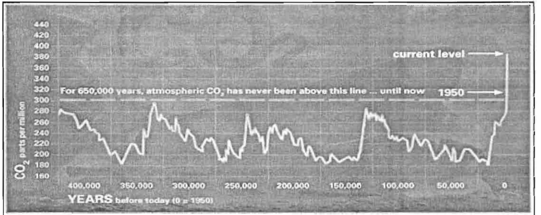
காபனீரொட்சைட்டின் அதிகரிப்பின் போக்கு
