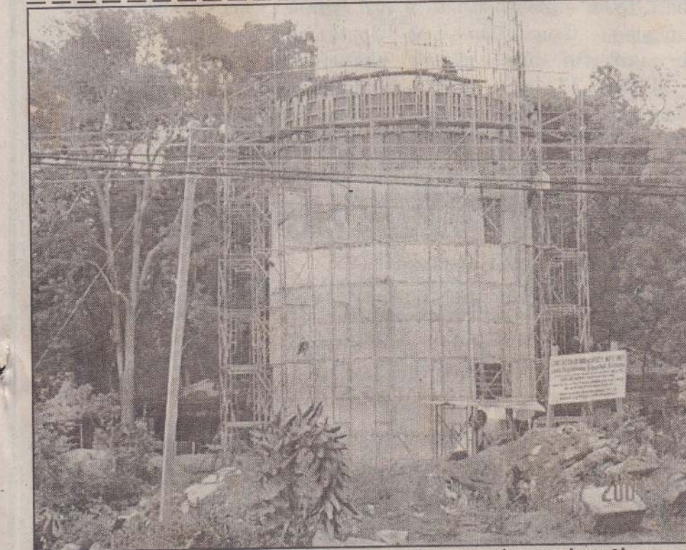
தேசிய நிர்வாககல் வடிகாலமைப்புச் சபையால் கிளிநொச்சி நகரப்பகுதிக்கான நீர் விநியோகத்திட்டத்திற்காக அமைக்கப்பட்டு வரும் நீர்த்தாங்கி வேலைகள் மிகவும் துரித கதியில் நடைபெற்று வருகின்றன. ஆயிரம் கன மீட்டர் கொள்ளளவுடைய கித்தாங்கி யுத்தத்தினால் ஏற்கனவே சேதமாகப்பட்ட தாங்கிக்கருகில் அமைக்கப்பட்டுவருவது குறிப்பிடத்தக்கது. புத்தாக அமைக்கப்படும் நீர்த்தாங்கியமைப்பதத்தில், காணலாம். (படம்: செந்தில்குமரன் - திருவையாறுச் செய்தியாளர்.)
