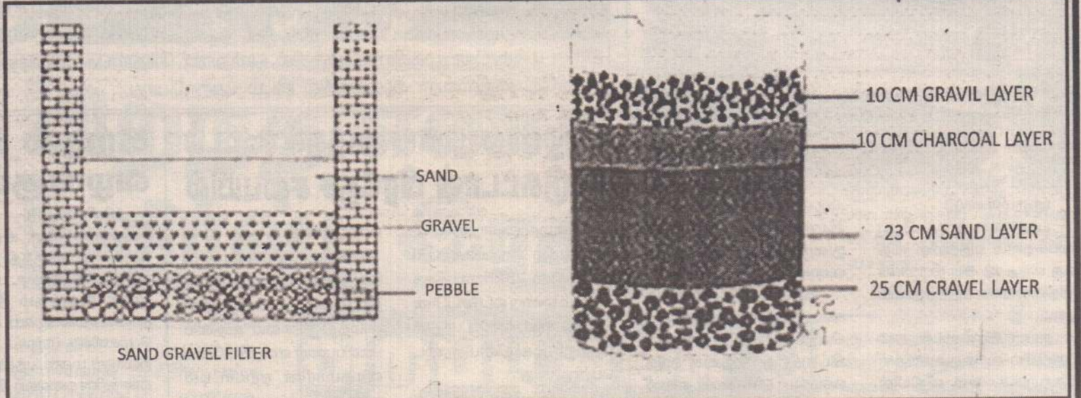
மணல், கிரவலைக் கொண்ட வடிகட்டும் தொகுதி
