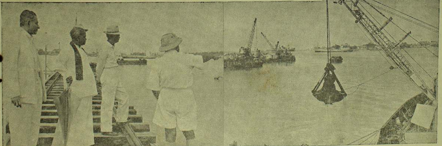
ஒரு கோடியே முப்பது லட்சம் ரூபா உத்தேசச் செலவில் கட்டப்படும் காலித்துறைமுகம் பூர்த்தியடைந்துவருகிறது. 1,400 அடி நீளமான அணையும் துறையினதும் 900 அடி அலைதாங்கியினதும் வேலை அநேகமாக முடிந்துவிட்டது. முழுவேலையும் அடுத்தவருடமுடிவுக்குள் பூர்த்தியாகிடுமென எதிர்பார்க்கப்படுகிறது.
