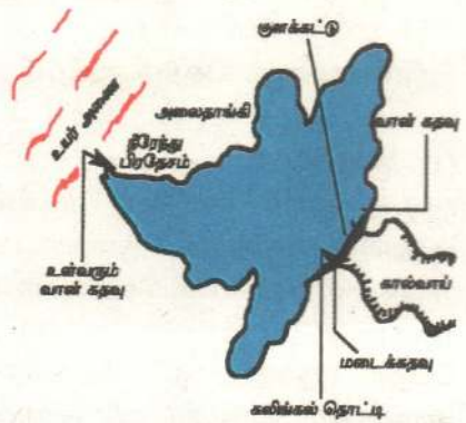
உரு 4.1 குளத்தின் பிரதான கூறுகள்.
