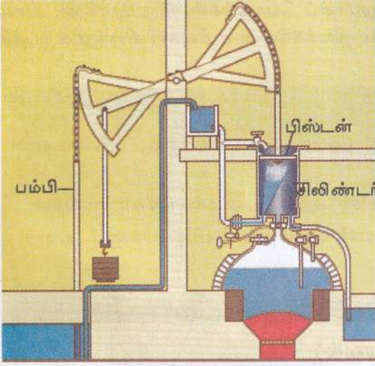
உரு 1.4 தோமஸ் நியூகொமனின் நீராவியால் இயங்கும் இயந்திரம்
