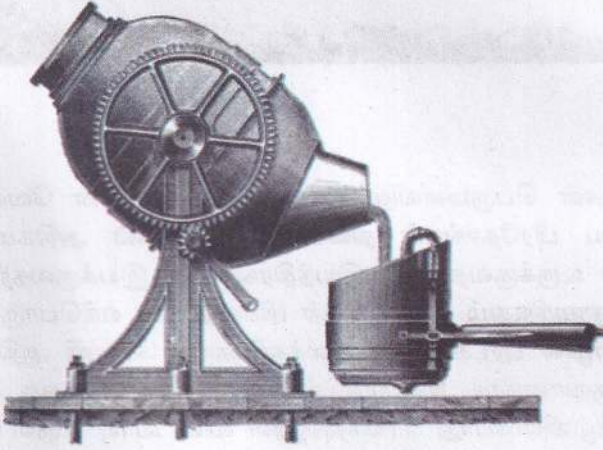
உரு 1.3 ஹென்றி பேஸ்மரின் உருக்கு உற்பத்தி உலை
