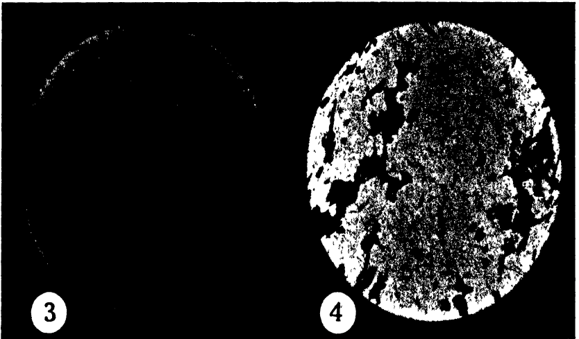
LEPTYNITES
