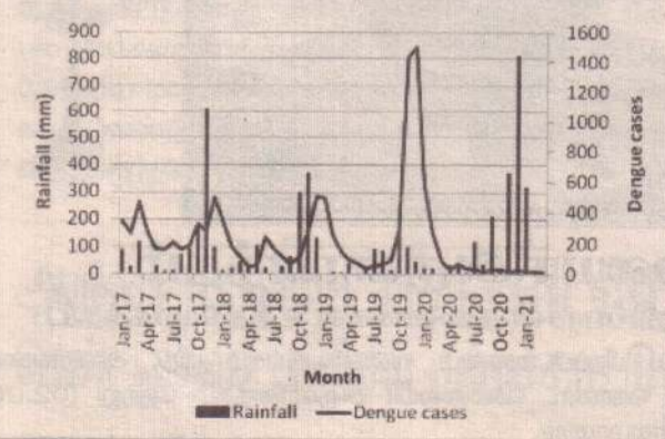
படம்-2: 2017-மார்ச் 2021 காலப்பகுதியில் யாழ் குடாநாட்டில் பதிவாகியுள்ள மாதாந்த மழை வீழ்ச்சி மற்றும் பெங்கு தொற்றாளர்கள்
