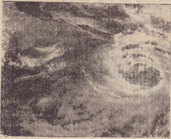
எல் - நைனோவின் விளைவால் பசுபிக் சமுத்திரக் கரையோரத்தின் மேல் உருவாகும் கரும்புயல், செயற்கைக் கோள் பிடித்த படம் இது.
